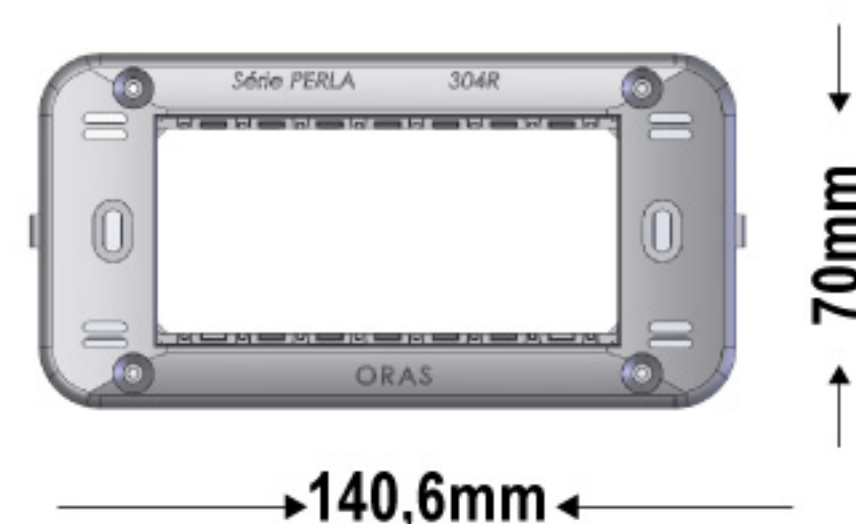
4 Módulos 304/RE
